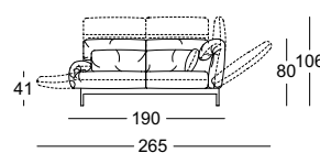
Gestofferde zitting
